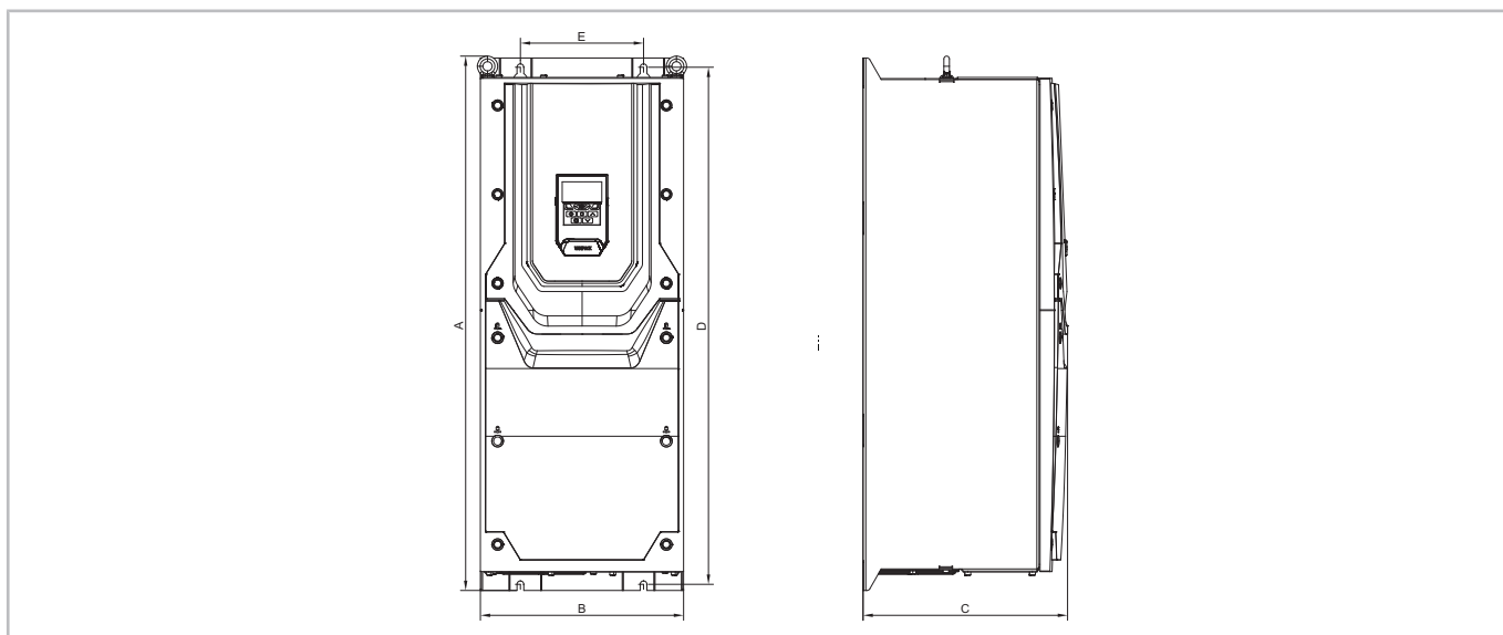
Fig. 6: IP55
