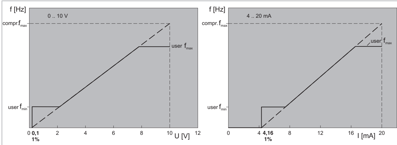
Abb. 10: Steuercharakteristik "0 .. Max"
