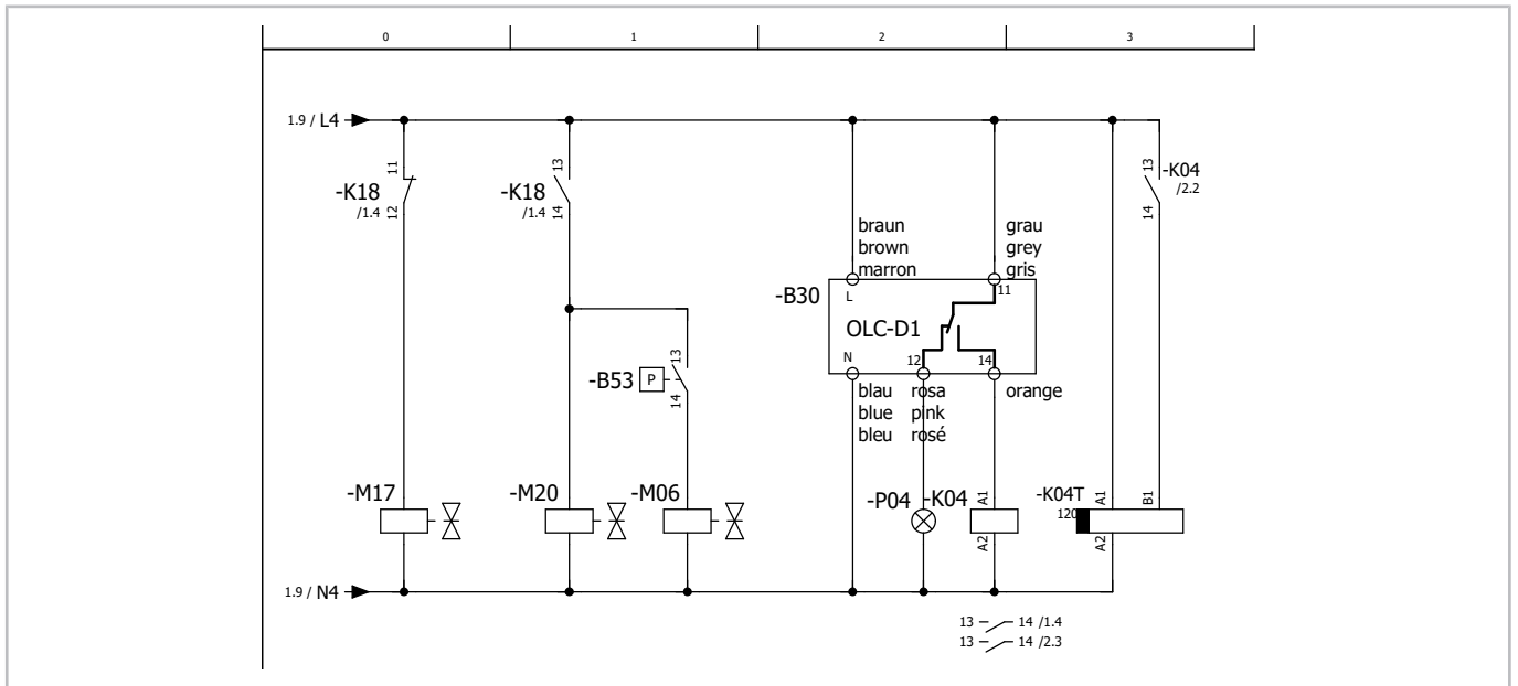
Abb. 17: Ölüberwachung HS.85-Schraubenverdichter
