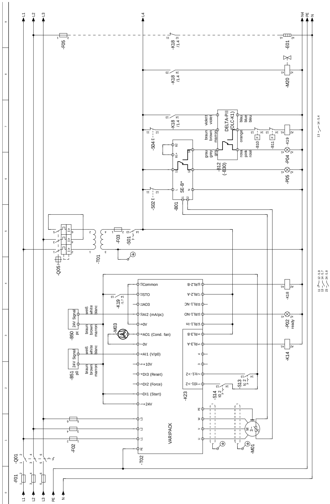
Abb. 13: Prinzipschaltbild Hubkolbenverdichter mit Erweiterungsmodul (K23)
