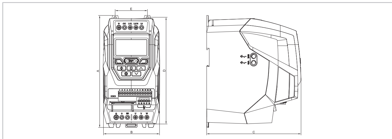
Fig. 4: IP20
