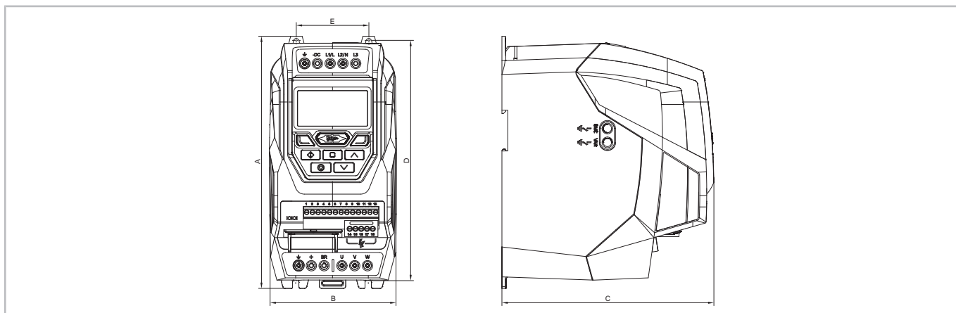
Abb. 4: IP20
