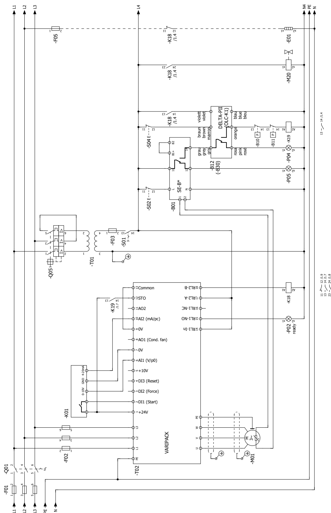
Abb. 12: Schaltbild Hubkolbenverdichter ohne Erweiterungsmodul
